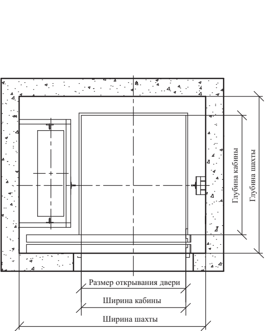
T1 План шахты
