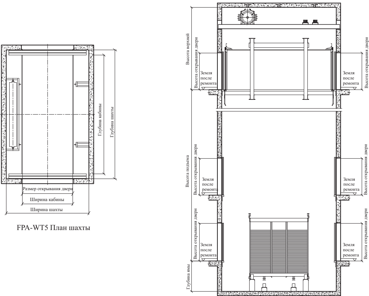
FPA-WT5 Вертикальный план шахты
