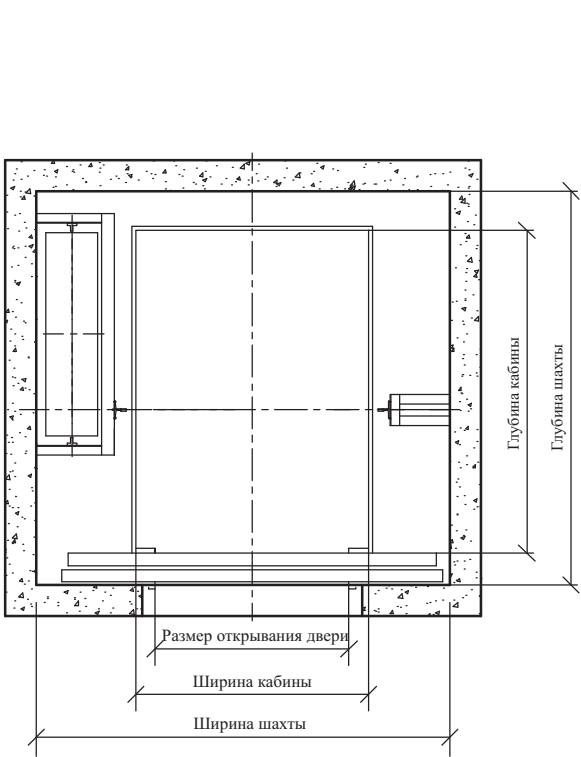
T3 План шахты
