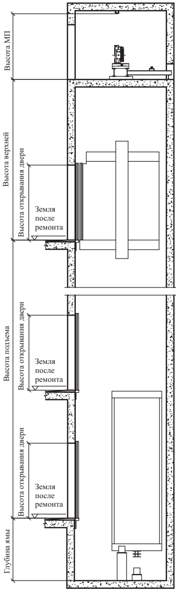
T3 Вертикальный план шахты
