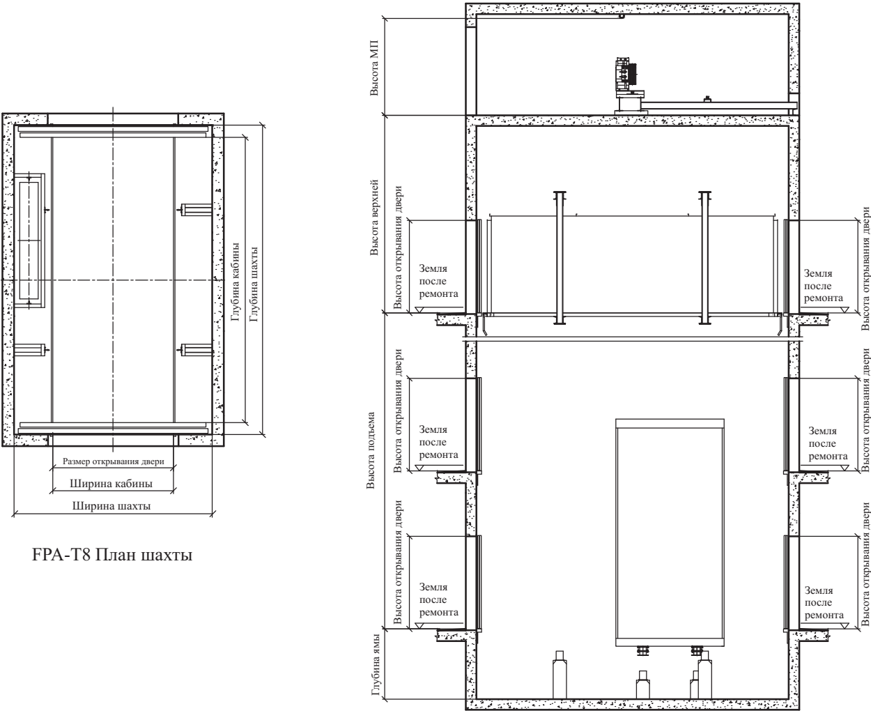
FPA-T8 Вертикальный план шахты
