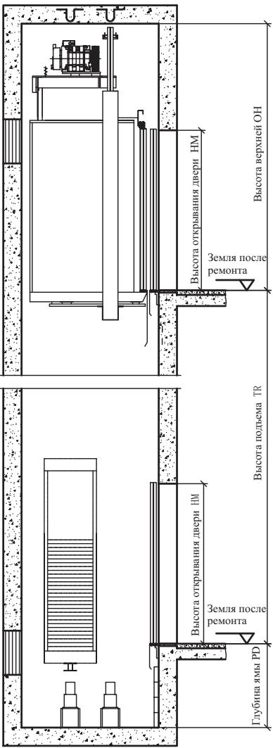
План шахты бокового открытия
