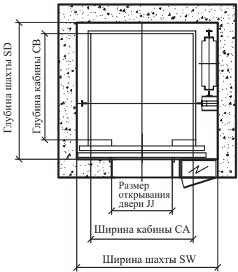
План шахты центрального открытия
